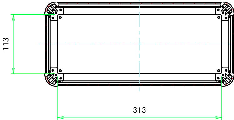
C-C ( 1 : 4.5 )
