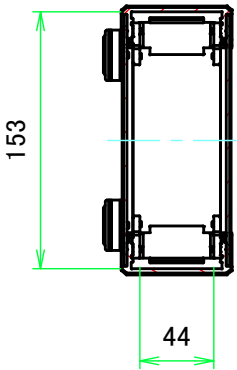
A-A ( 1 : 4.5 )
